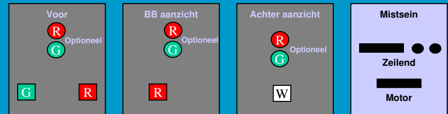
Regel 26 Vissersboten
